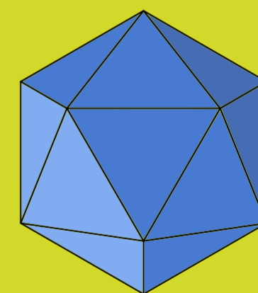
icosaedro
