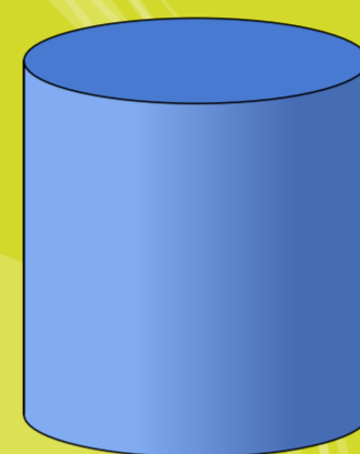
cilindro
