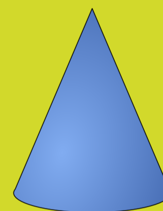
cono
