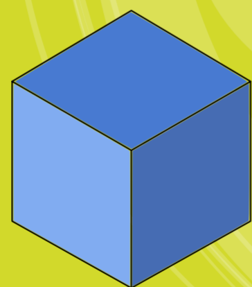
cubo
