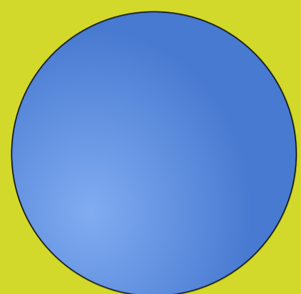
esfera
