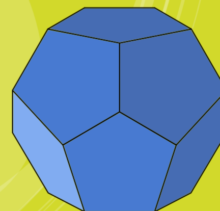
dodecaedro
